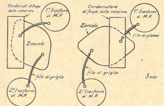
Fig. 3. - A sinistra: cattiva disposizione della valvola che può determinare effetto rigenerativo. - A destra: disposizione razionale.
