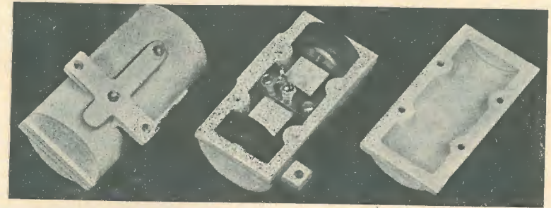
Fig. 5. - Elementi del filtro a cristallo a tre elettrodi. Queste lamine di quarzo hanno terminali in rame e sono montate nell'interno di una incastellatura fusa in alluminio che
